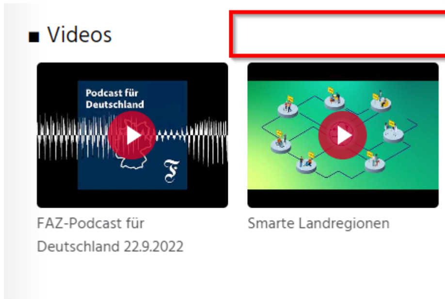
Abbildung 3 Startseite – Video-Paginierung
