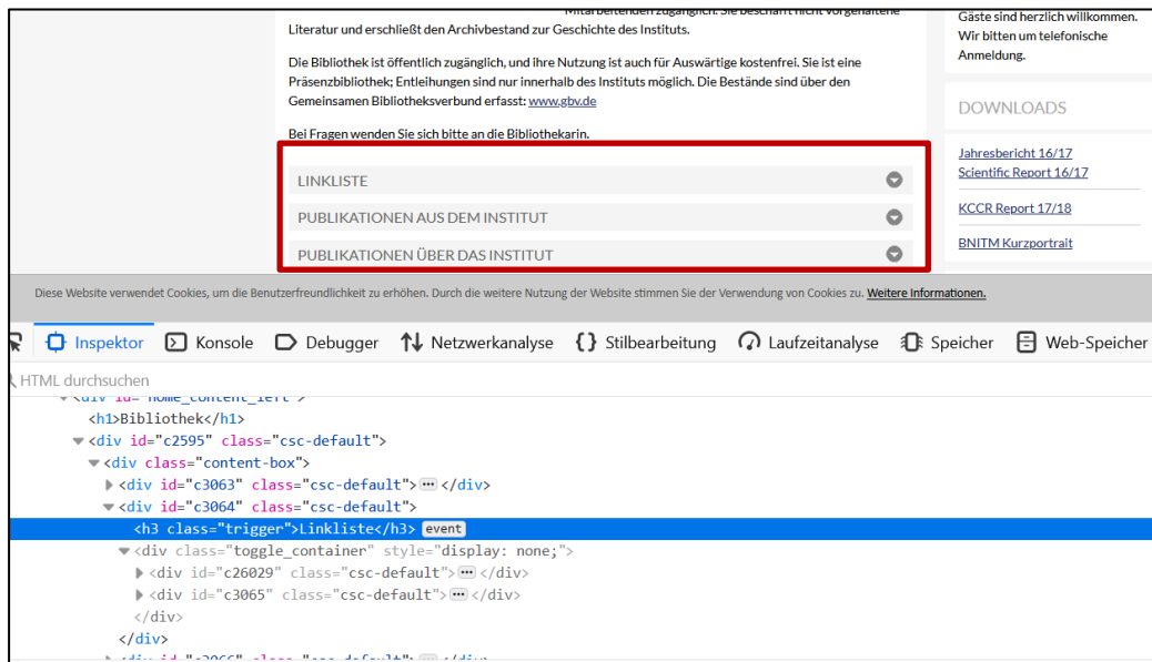
Abbildung 33: Akkordeon-Modul auf der Seite „Bibliothek“
