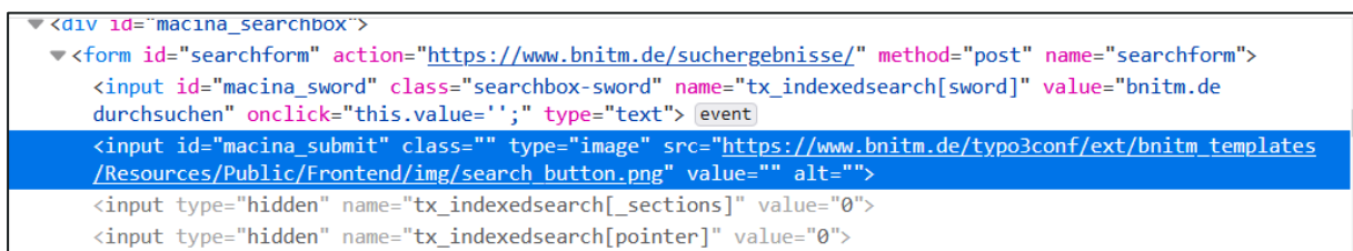
Abbildung 2: Quelltext Suchen-Schalter im Kopfbereich
